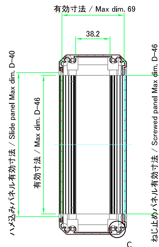
B-B ( 1 : 2.5 )
